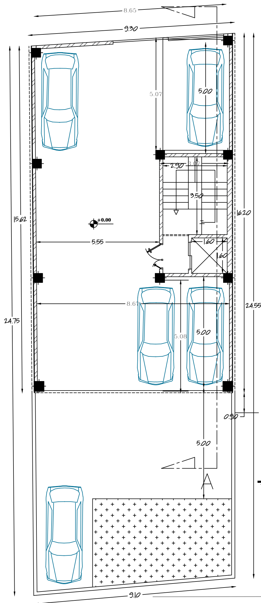
پلان هم کف Scale : 1 \ 100
